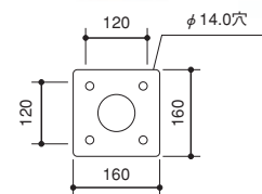
板厚 9 台板・受板
